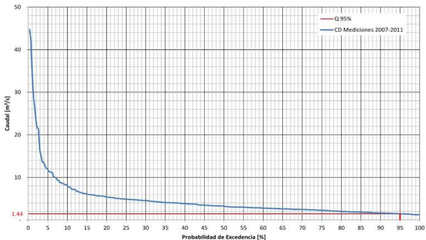
Curva de duración en sitio de toma RF
